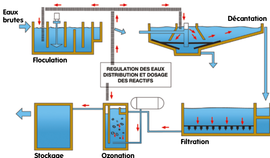
Les étapes du traitement de l'eau
